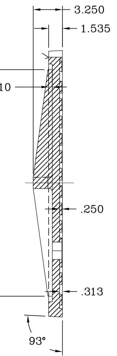
SECTION A-A
