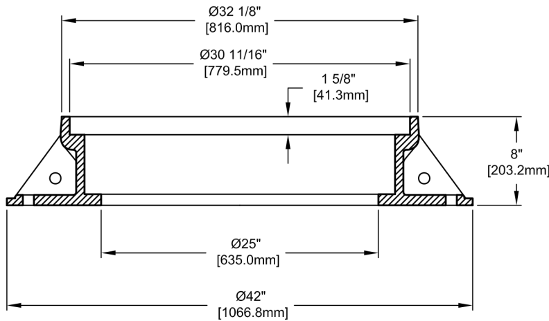
Cadre
