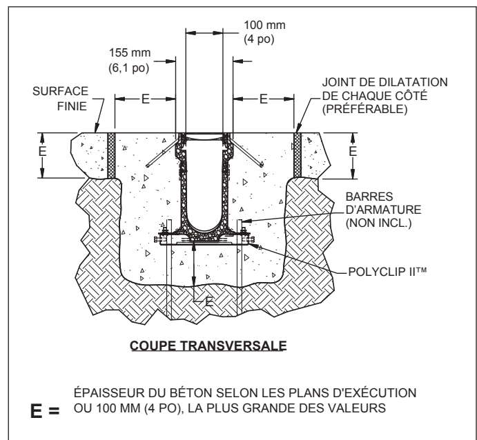
Barres d'armature
